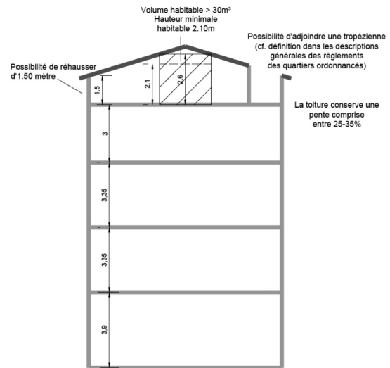
Exemple d'une construction en R+3 + combles
